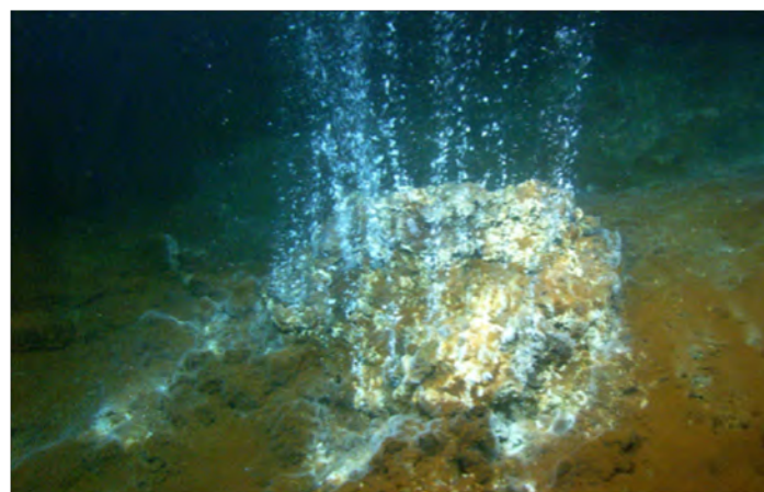
Tiefseethermalquelle n
